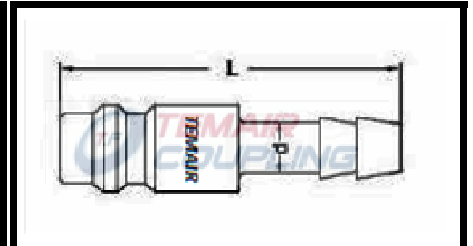
HORTUM UÇ
