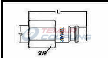
DIŞİ UÇ
