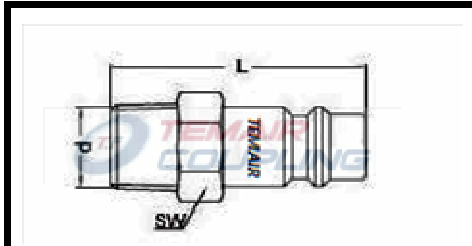
ERKEK UÇ
