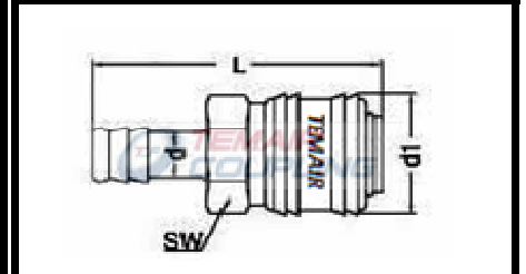
HORTUM GÖVDE
